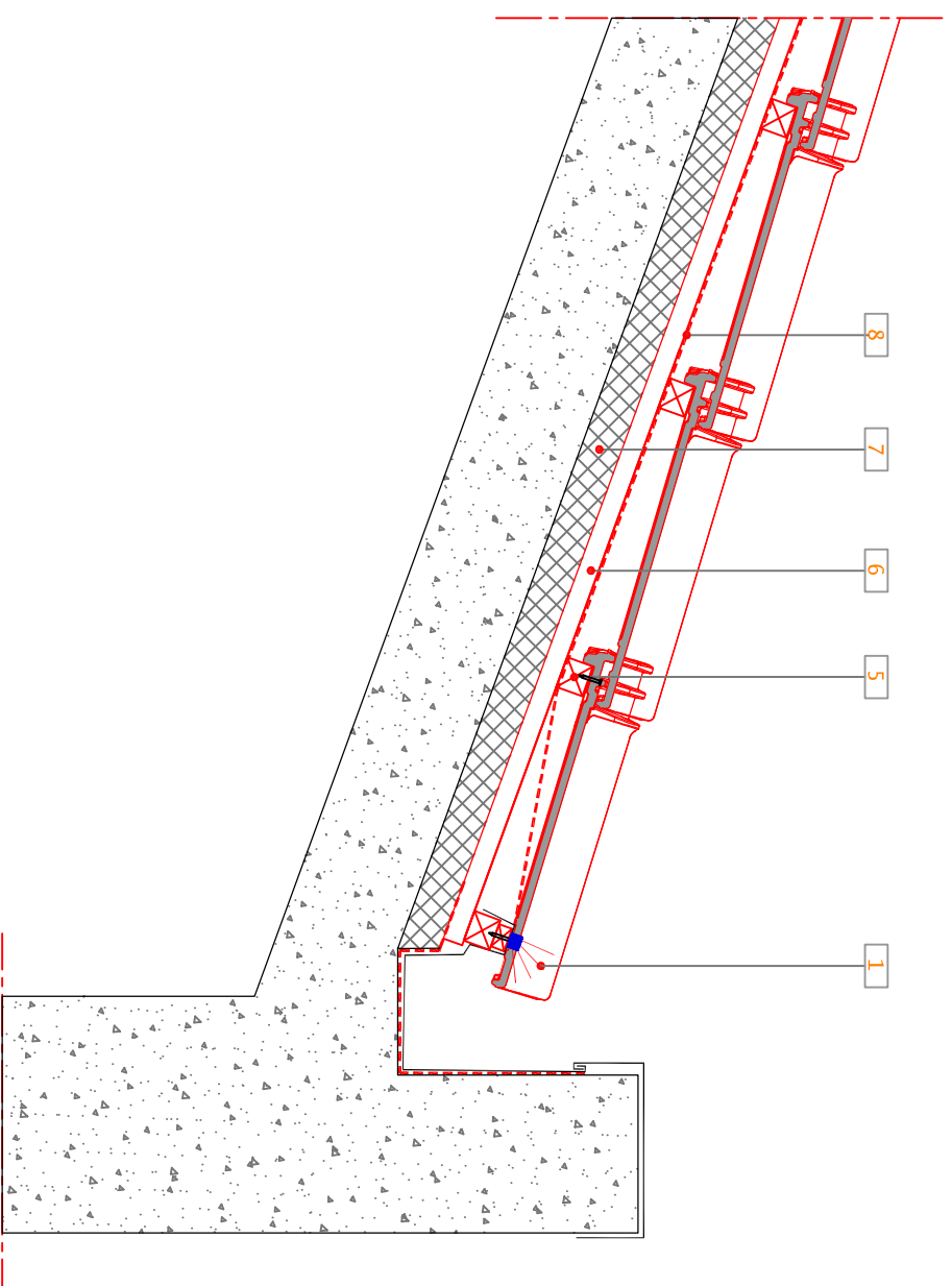
161 Corte vertical transversal - Pormenor ripado + contra-ripado
