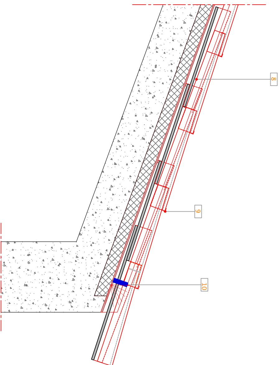
322 Corte vertical transversal - Pormenor com subtelha UM placa 190
