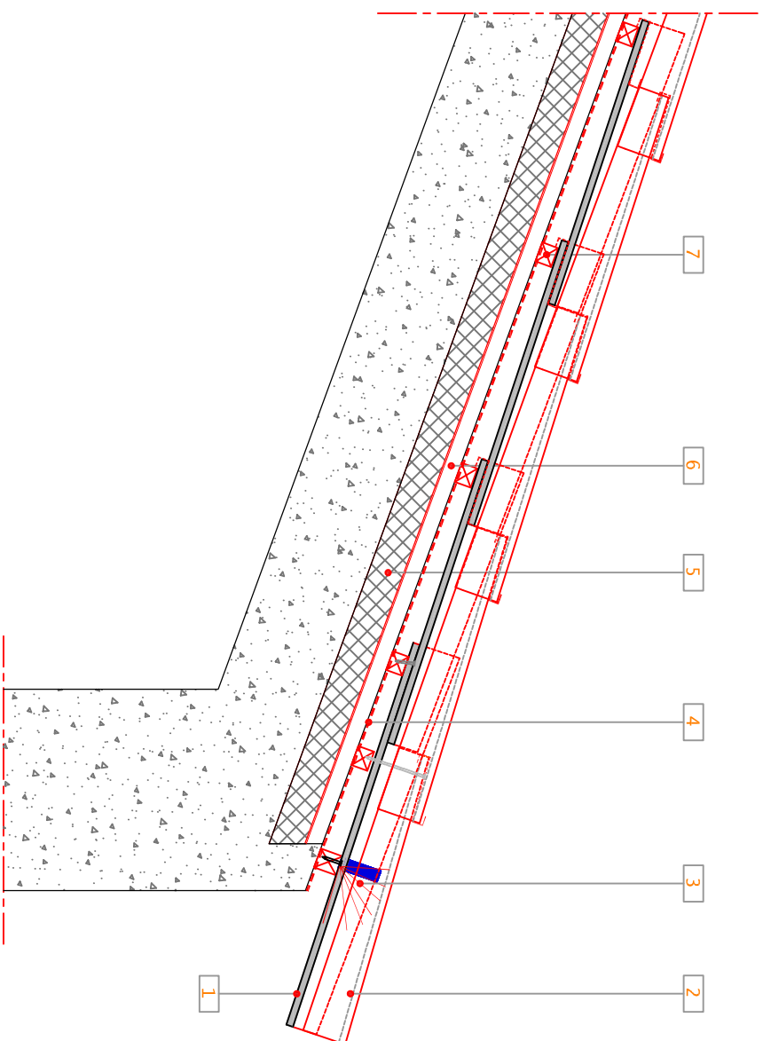
321 Corte vertical transversal - Pormenor ripado e contra-ripado
