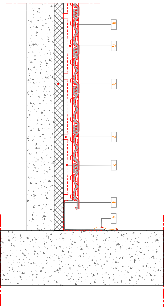
281 Corte vertical [longitudinal] - Pormenor ripado + contra-ripado
