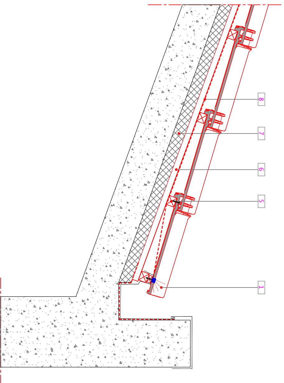
161 Corte vertical transversal - Pormenor ripado + contra-ripado
