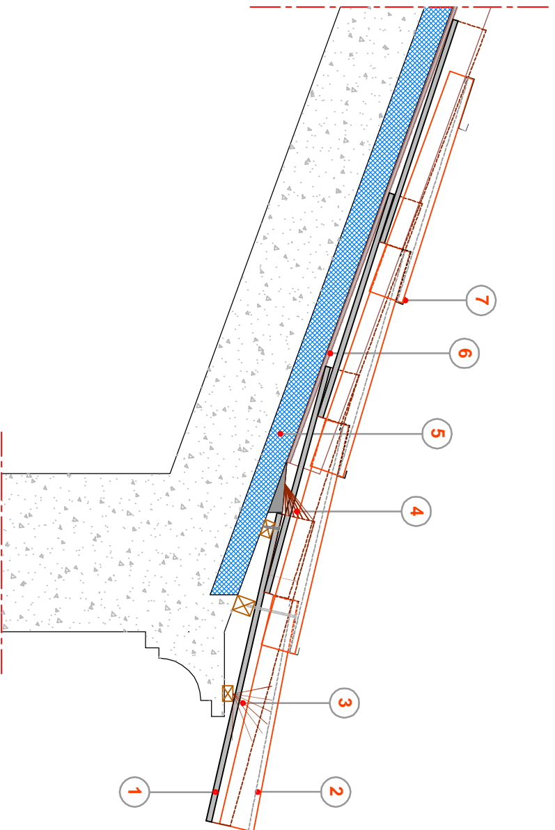
Pormenor com sub-telha UM placa 190
